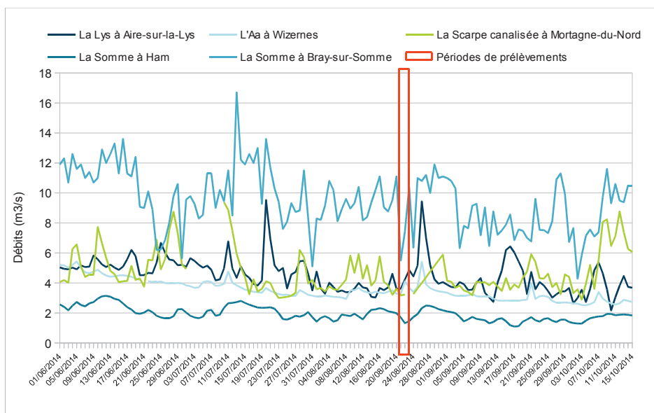
Figure 7: Débits journaliers observés sur les grands cours d'eau du bassin versant Artois-Picardie – juin à octobre 2014 - (Données HYDRO/MEDD/DE)
