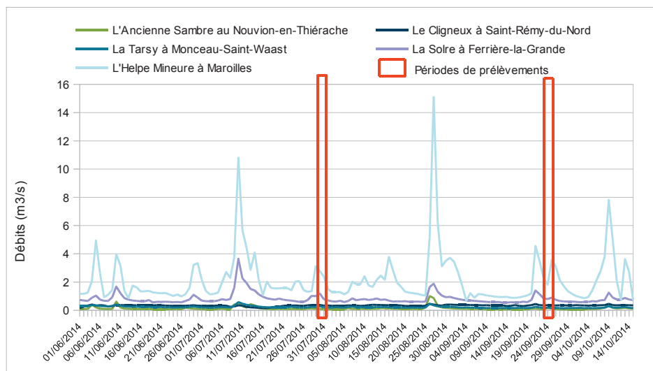
Figure 6: Débits journaliers observés sur le bassin versant de la Sambre – juin à octobre 2014 - (Données HYDRO/MEDD/DE)
