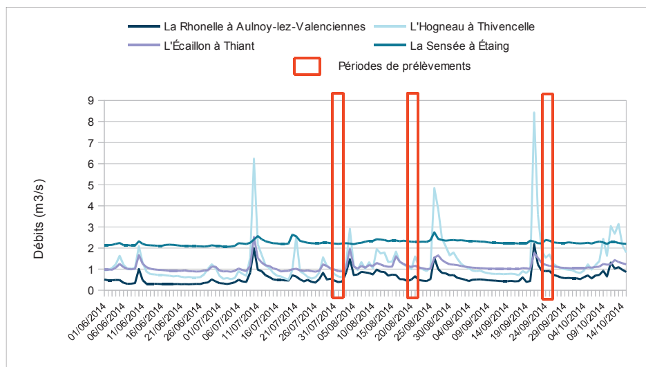
Figure 5: Débits journaliers observés sur le bassin versant Scarpe/Escaut – juin à octobre 2014 - (Données HYDRO/MEDD/DE)
