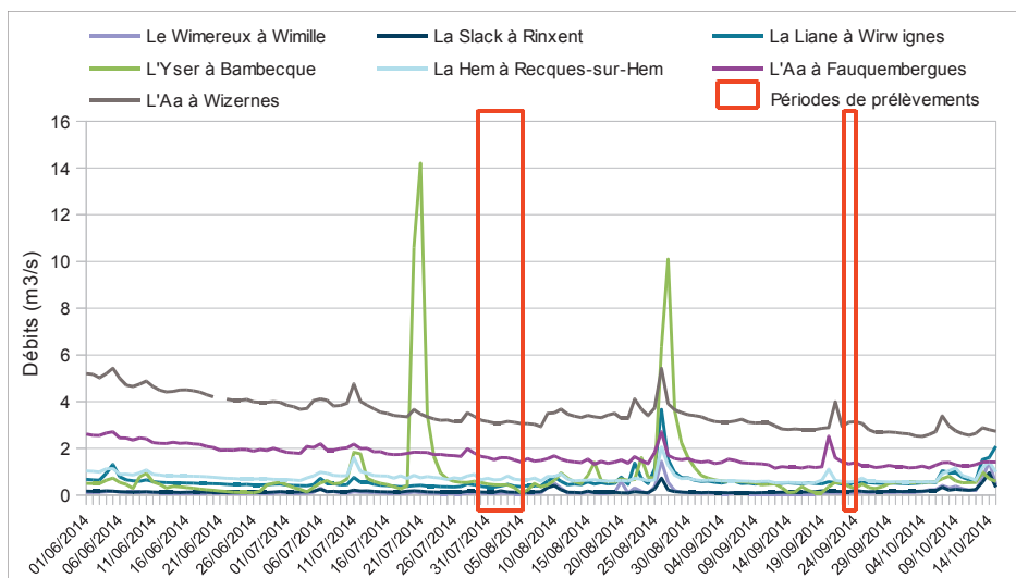
Figure 3: Débits journaliers observés sur les cours d'eau côtiers du Nord – juin à octobre 2014 - (Données HYDRO/MEDD/DE)
