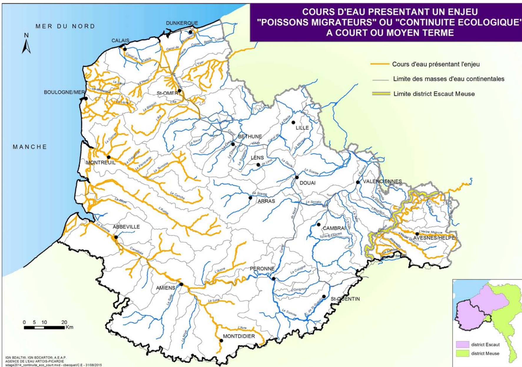
Carte 19 : Cours d'eau présentant un enjeu "poissons migrateurs" ou "continuité écologique" à court ou moyen terme
