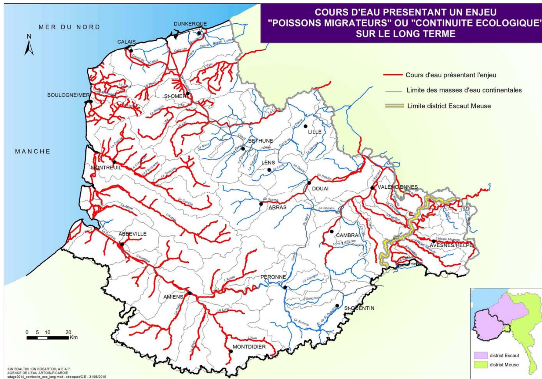
Carte 18 : Cours d'eau présentant un enjeu "poissons migrateurs" ou "continuité écologique" sur le long terme
