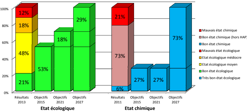
Figure 7 : Etat et objectifs du SDAGE 2010-2015 des cours d'eau
