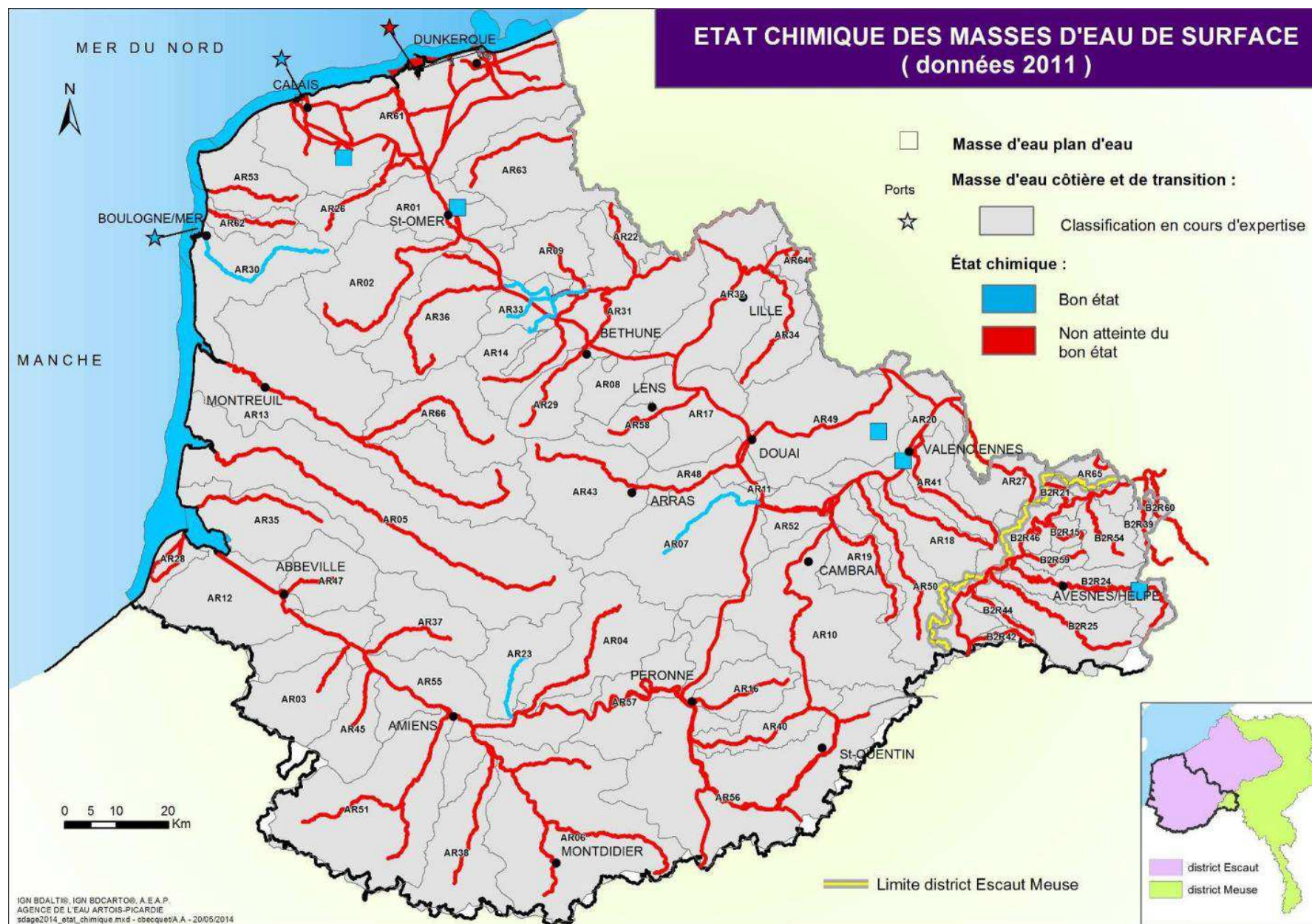
Carte 26 : Etat chimique des masses d'eau de surface (données 2011)
