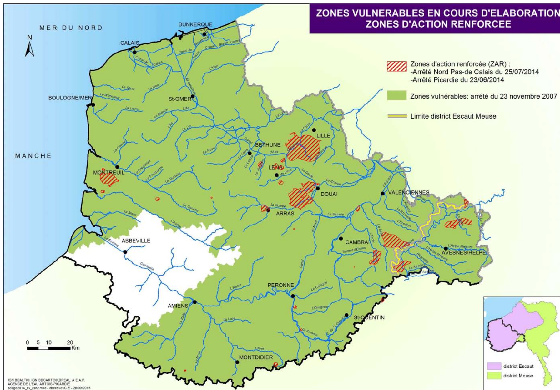
Carte 23 : Zones vulnérables en cours d'élaboration - Zones d'action renforcée
