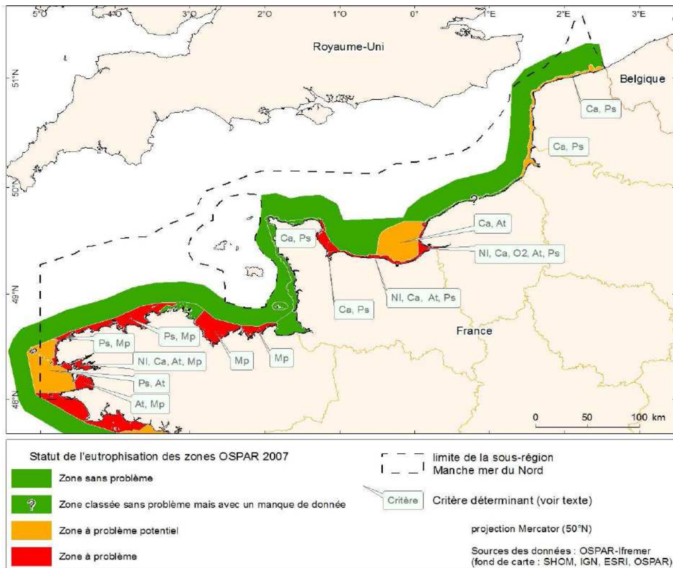
Carte 34 : Résultat du classement des zones OSPAR de la sous-région marine Manche Mer du Nord par la mise en œuvre de la procédure commune d'évaluation de l'eutrophisation, en 2007
