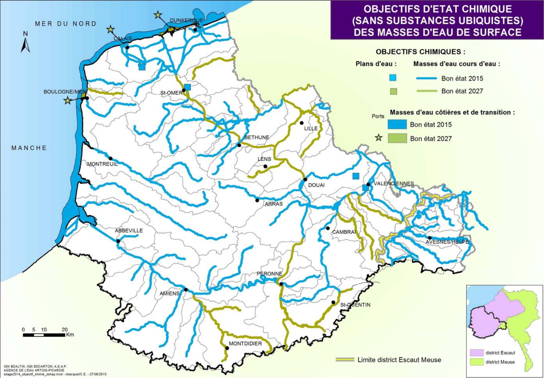
Carte 9 : Objectifs d'état chimique (sans substances ubiquistes) des masses d'eau de surface
