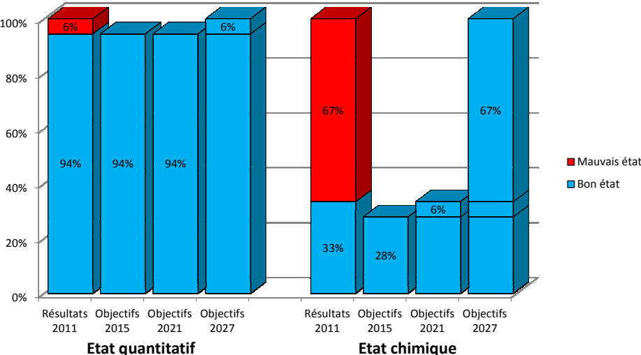
Figure 6 : Etat et objectifs du SDAGE 2010-2015 des eaux souterraines
