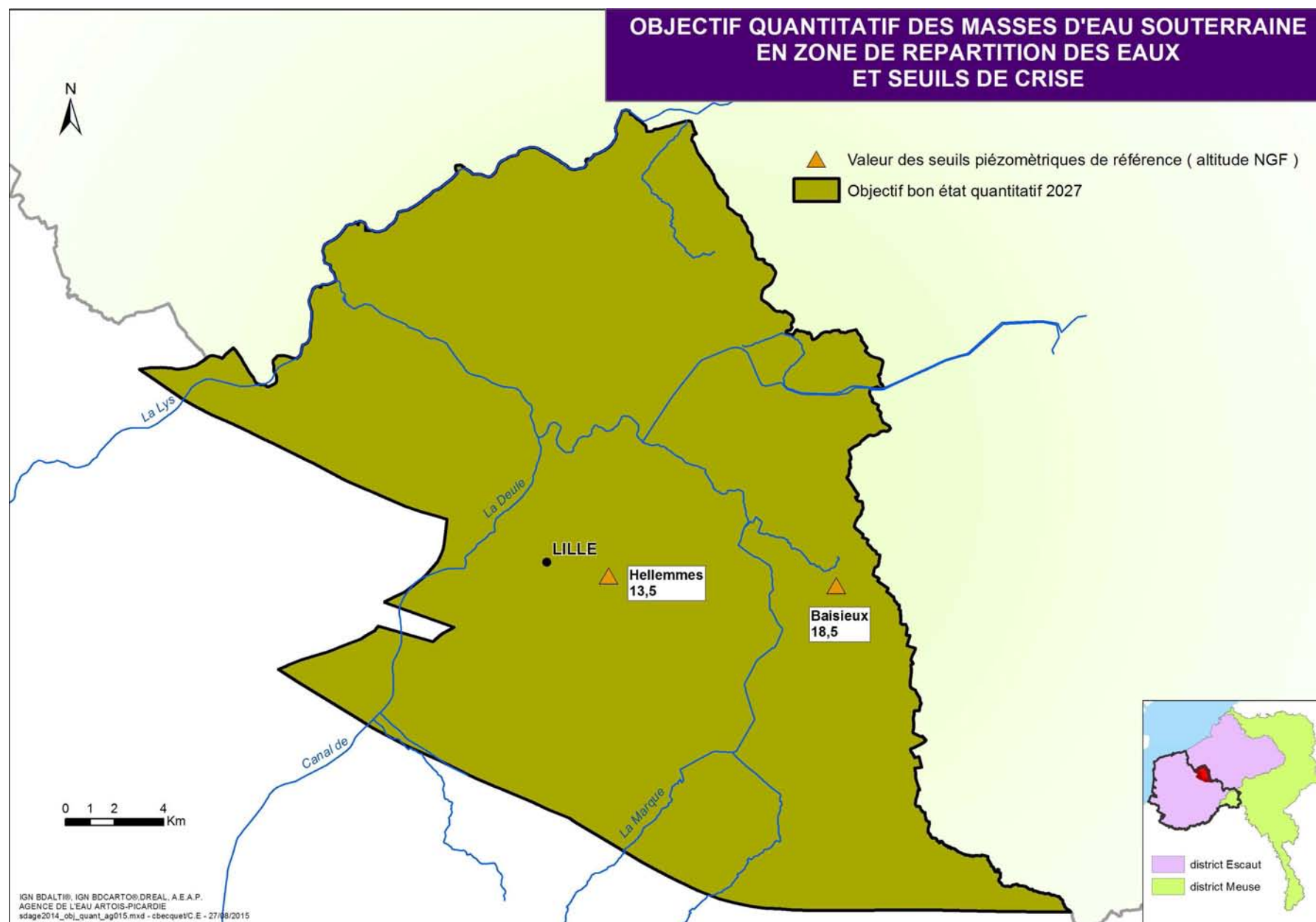
Carte 14 : Objectifs d'état quantitatif des masses d'eau souterraine en zone de répartition des eaux et seuils de crise
