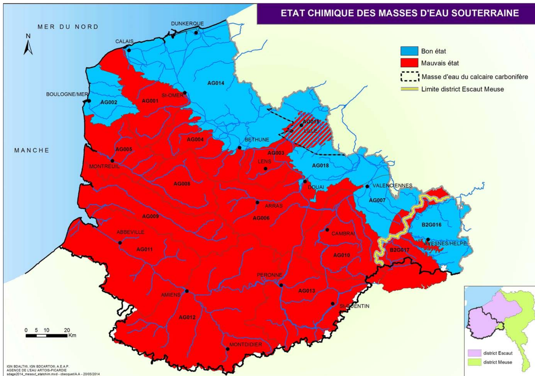
Carte 30 : Etat chimique des masses d'eau souterraine
