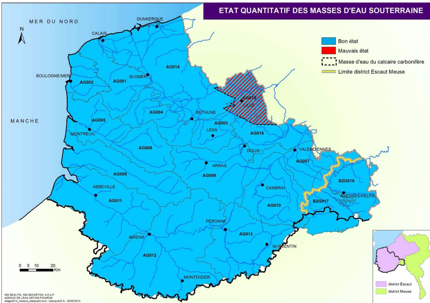
Carte 29 : Etat quantitatif des masses d'eau souterraine
