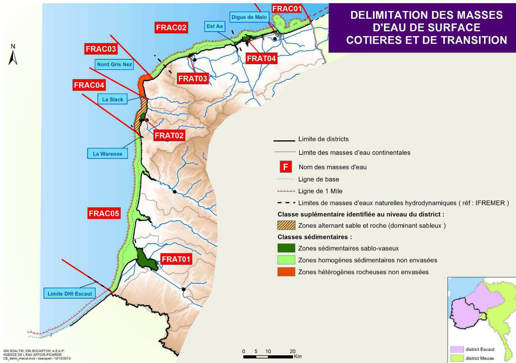
Carte 4 : Délimitation des masses de surface côtières et de transition
