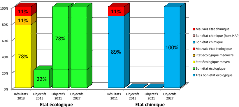
Figure 9 : Etat et objectifs du SDAGE 2010-2015 des eaux littorales
