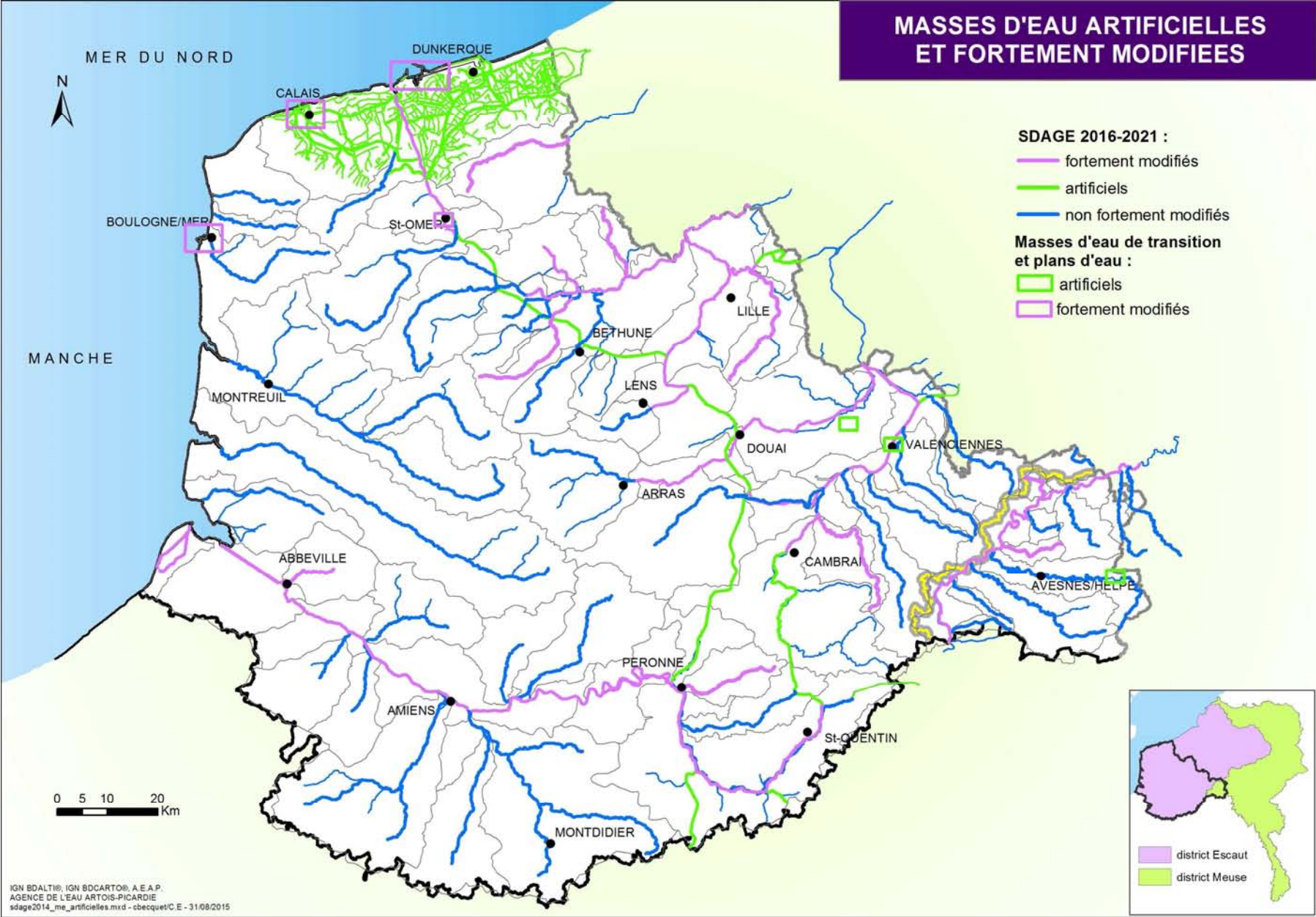
Carte 6 : Masses d'eau artificielles et fortement modifiées
