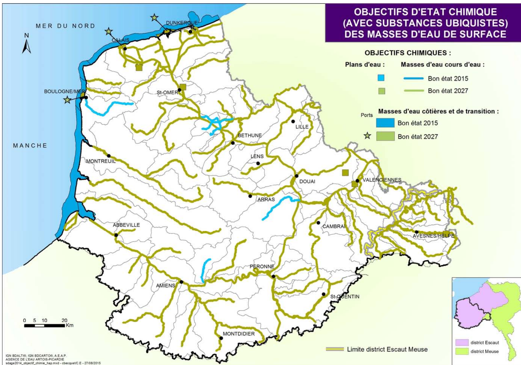
Carte 8 : Objectifs d'état chimique (avec substances ubiquistes) des masses d'eau de surface
