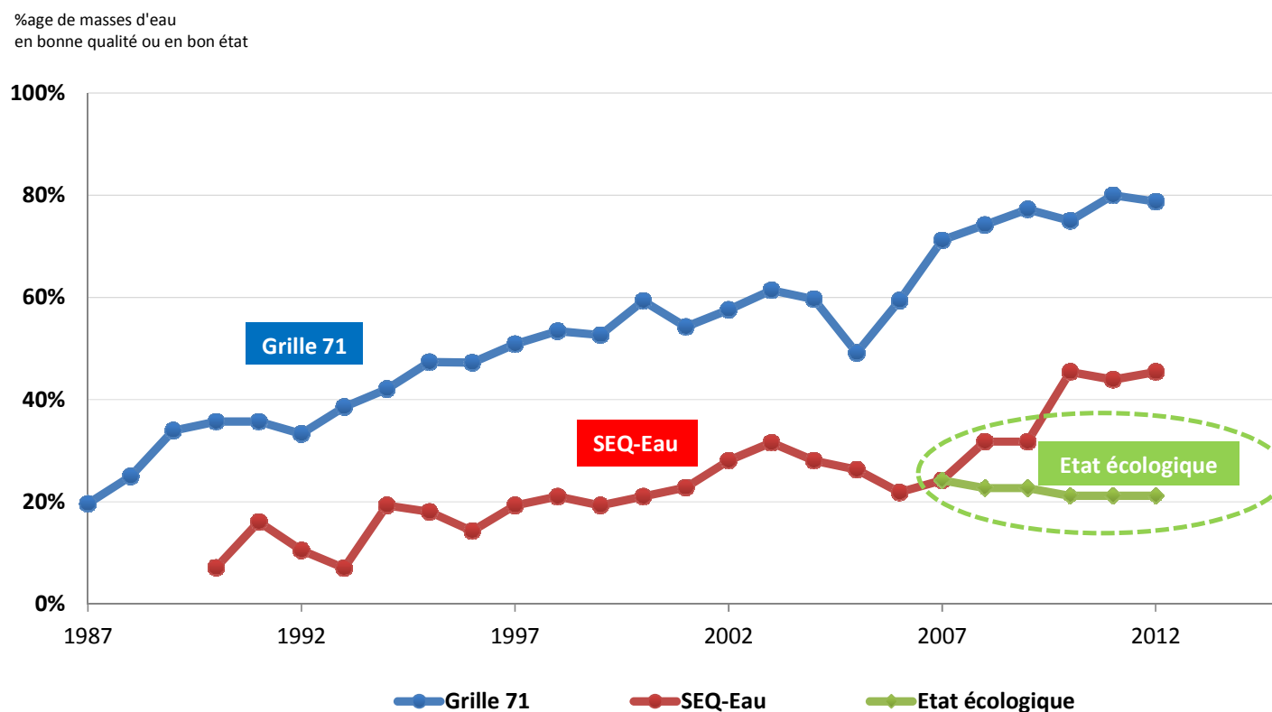
Figure 10 : Evolution depuis 1987 du pourcentage de masses d'eau en classe de qualité "bon" selon les 3 systèmes d'évaluation
