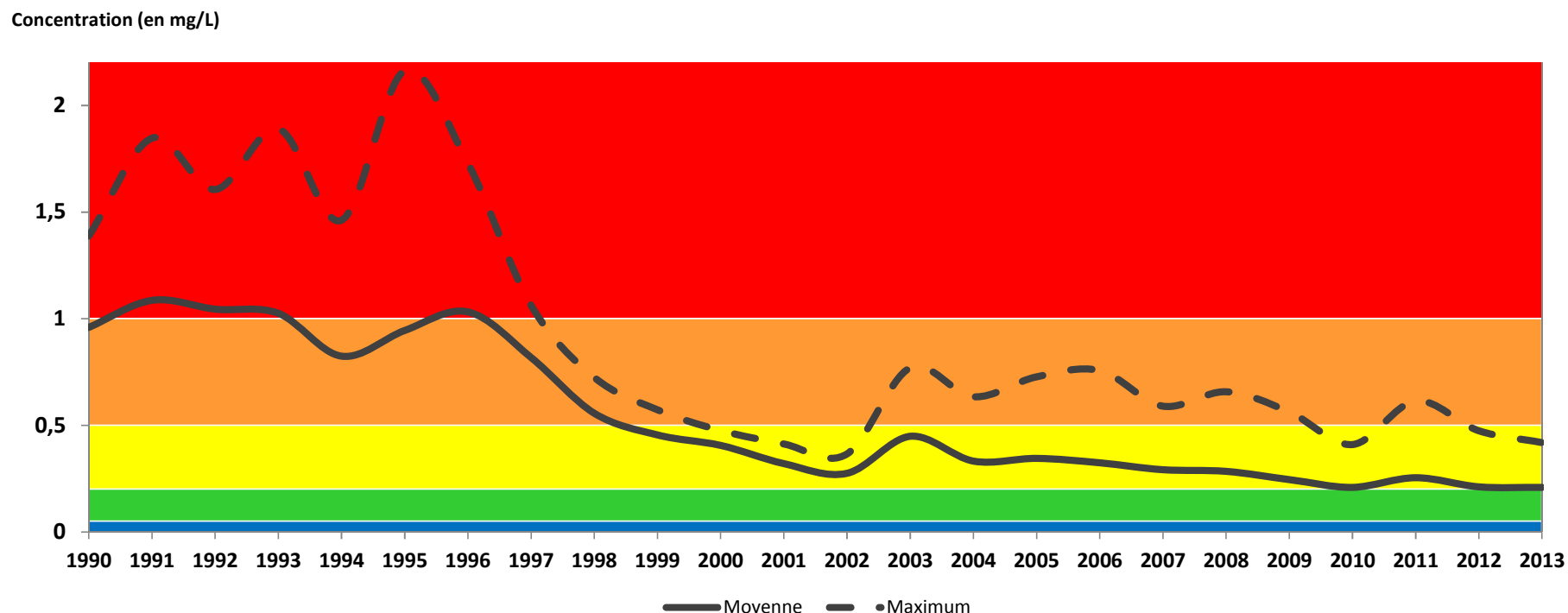
Figure 11 : Evolution des concentrations moyennes et maximales en phosphore sur les cours d'eau du bassin
