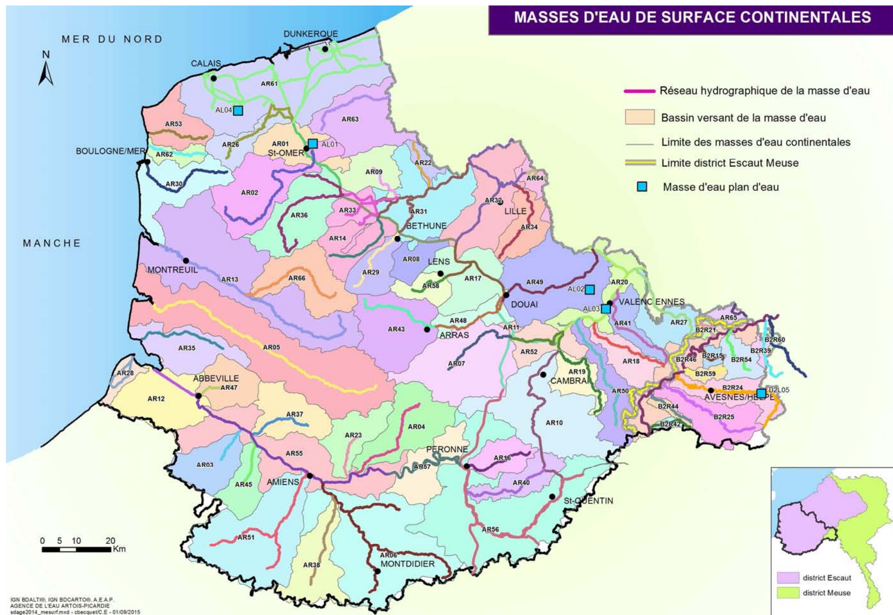
Carte 3 : Masses d'eau de surface continentales
