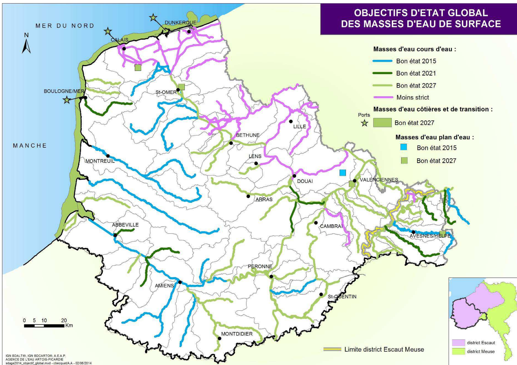
Carte 10 : Objectifs d'état global des masses d'eau de surface
