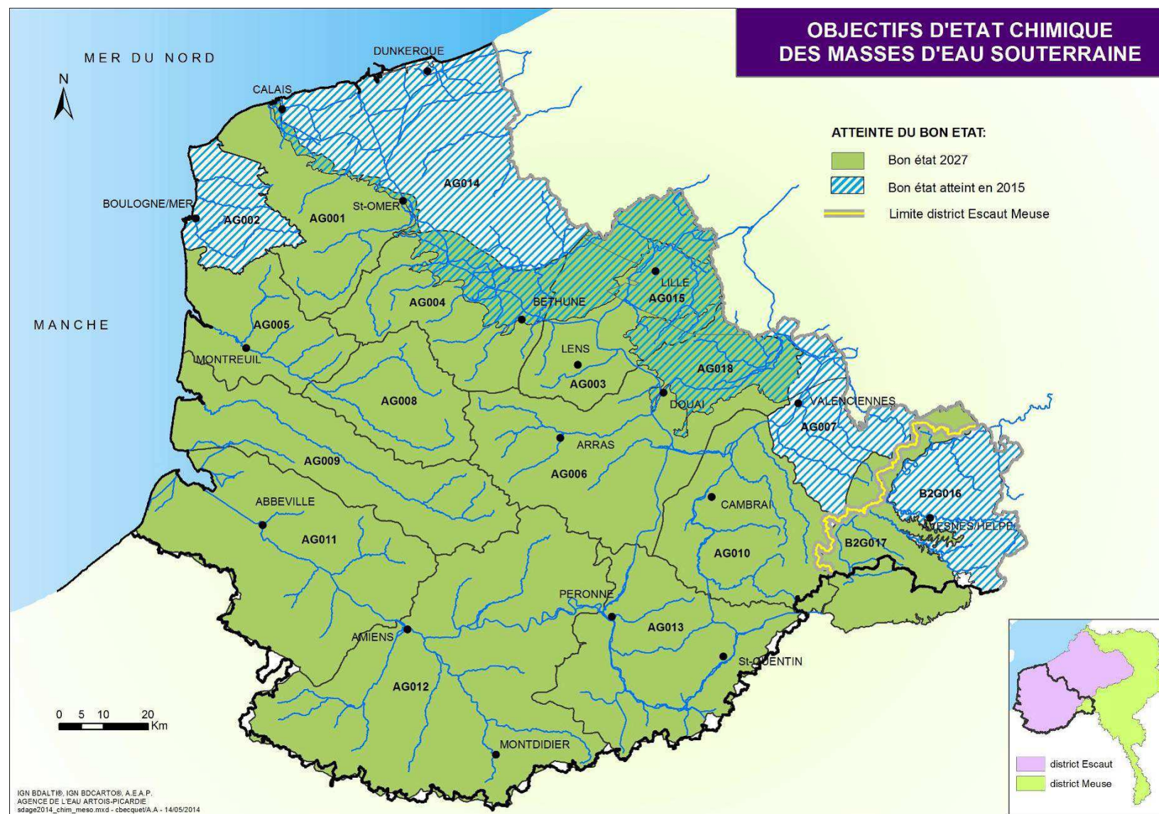
Carte 11 : Objectifs d'état chimique des masses d'eau souterraine
